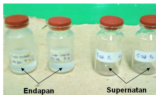
Gambar 2. Pemisahan endapan ^{137}CsClO_4 dengan supernatan
