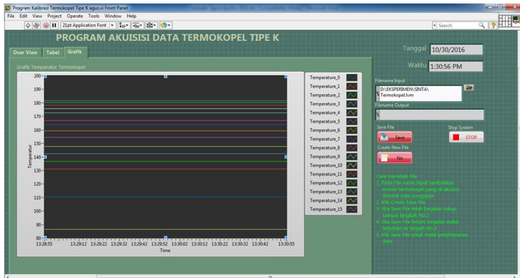
Gambar 10. Tampilan antarmuka akuisisi data termokopel tipe K dalam bentuk grafik
