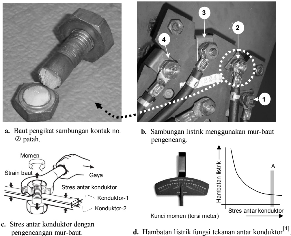
Gambar 6. Pengencangan mur-baut berlebihan berpotensi merusak.
