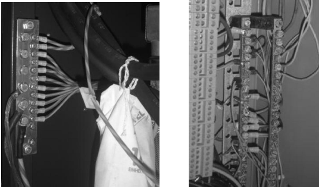
Gambar 4. (a) Tidak ada jamur tumbuh di terminal kabel karena penempatan zat higroskopis dalam kabinet perangkat. (b) Jamur tumbuh di terminal kabel akibat tidak ada zat higroskopis dalam kabinet perangkat.
