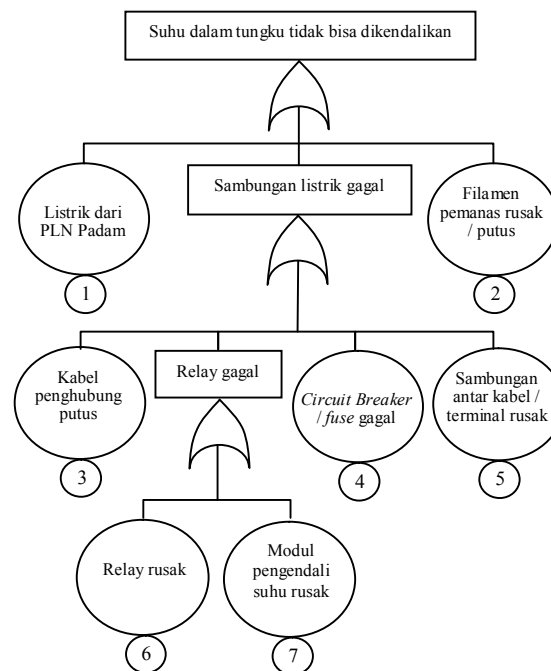
Gambar 7. Bagan FTA gagalnya pengendalian suhu
