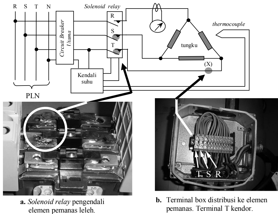
Gambar 5. Sambungan jelek sumber di/dt berulang pada perangkat tungku pemanas.
