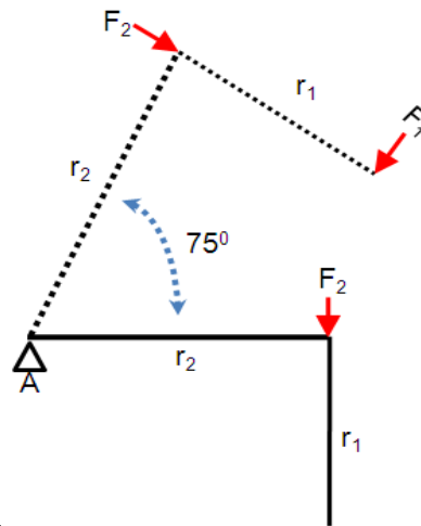
Gambar 3. Diagram Pembebanan Rangka Sandaran Kursi
