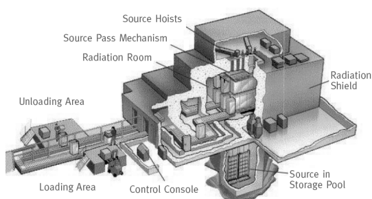
Gambar.4. Gambar skema instalasi iradiator gamma untuk pengawetan hasil pertanian atau produk olahannya/ makanan [11]
