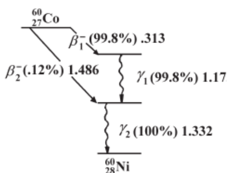
Gambar. 3. Skema peluruhan sumber radioaktif Cobalt-60
