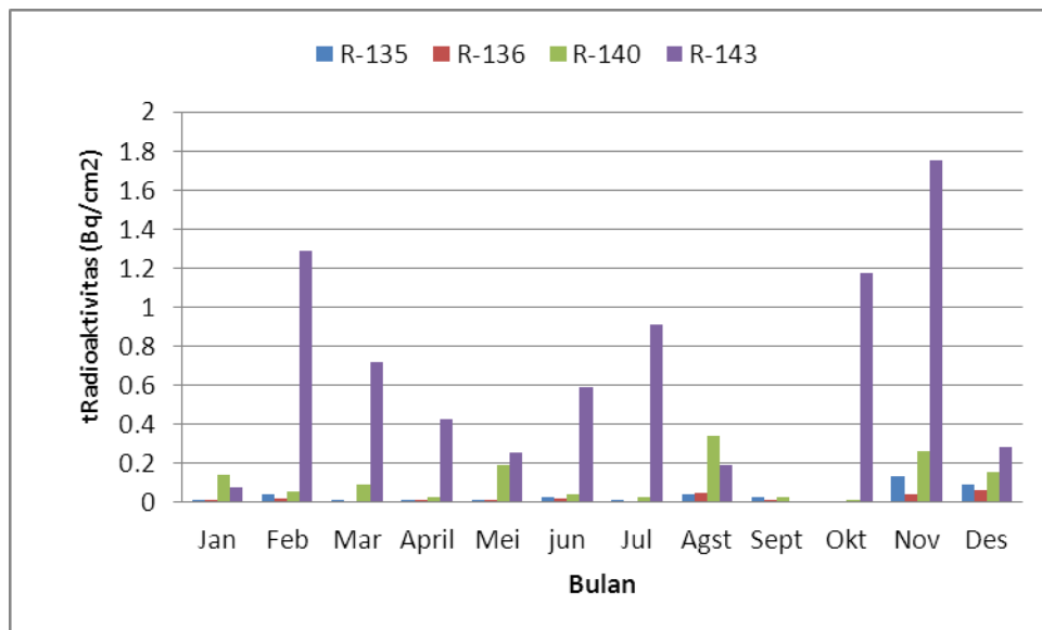
Gambar 5. Radioaktivitas \beta permukaan lantai Gedung IRM tahun 2018
