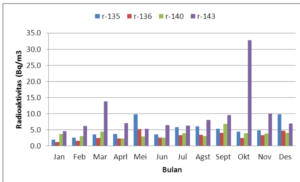
Gambar 3. Radioaktivitas β udara Gedung IRM tahun 2018
