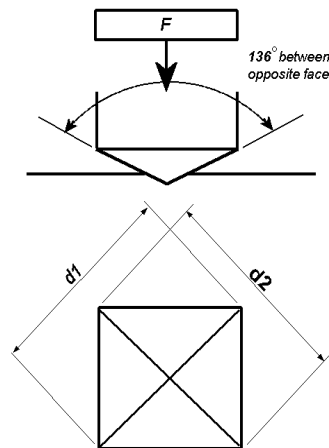
Gambar-1. Metode uji kekerasan model vickers
