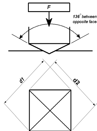
Gambar-1. Metode uji kekerasan model vickers
