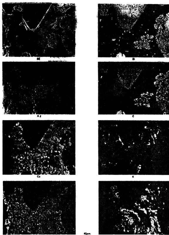
Gambar 7. Hasil analisa hard spot yang menunjukkan jumlah unsur pada logam cor aluminium
