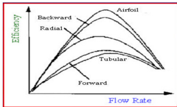
Gambar 2. Efisiensi versus laju alir
