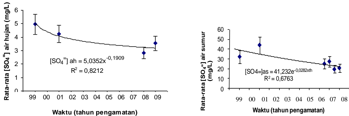
Gambar 3. Pola perubahan kadar \text{SO}_4^- dalam air hujan (a) dan kadar \text{SO}_4^- dalam air sumur (b) pada daerah yang sering mengalami hujan asam intensitas tinggi di wilayah industri Cibinong-Citeureup Kabupaten Bogor ( error bar 15% dan 20%).
