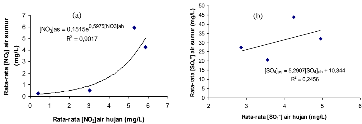
Gambar 4. Hubungan kadar nitrat dalam air hujan terhadap kadar nitrat dalam air sumur (a) dan hubungan antara kadar sulfat dalam air hujan dan air sumur (b) pada daerah yang sering mengalami hujan asam intensitas tinggi di wilayah industri Cibinong-Citeureup kabupaten Bogor.
