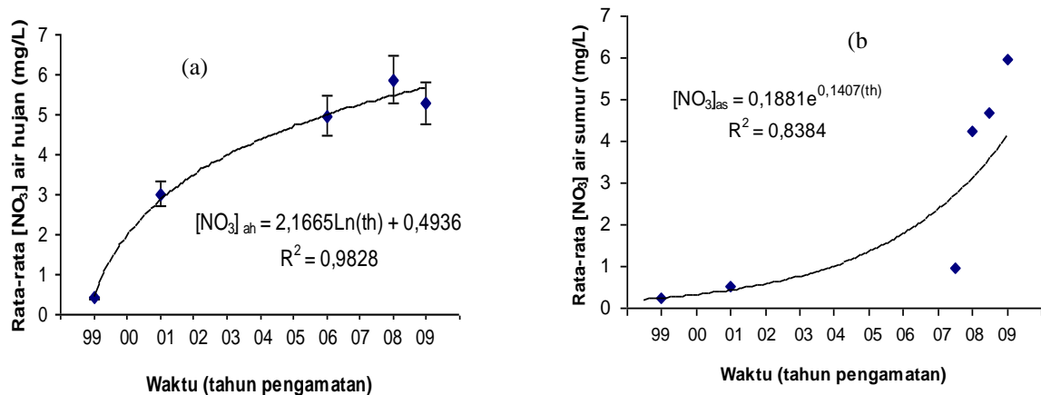
Gambar 2. Kecenderungan rata-rata perubahan kadar nitrat dalam air hujan (a) ( error bars 10%) dan pola perubahan kadar nitrat dalam air sumur (b) pada daerah yang sering mengalami hujan asam intensitas tinggi di wilayah industri Cibinong-Citeureup Kabupaten Bogor.
