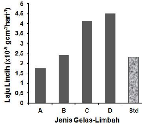
Gambar 3. Pengaruh Jenis Gelas-Limbah Terhadap Laju Pelindihan Gelas-Limbah
