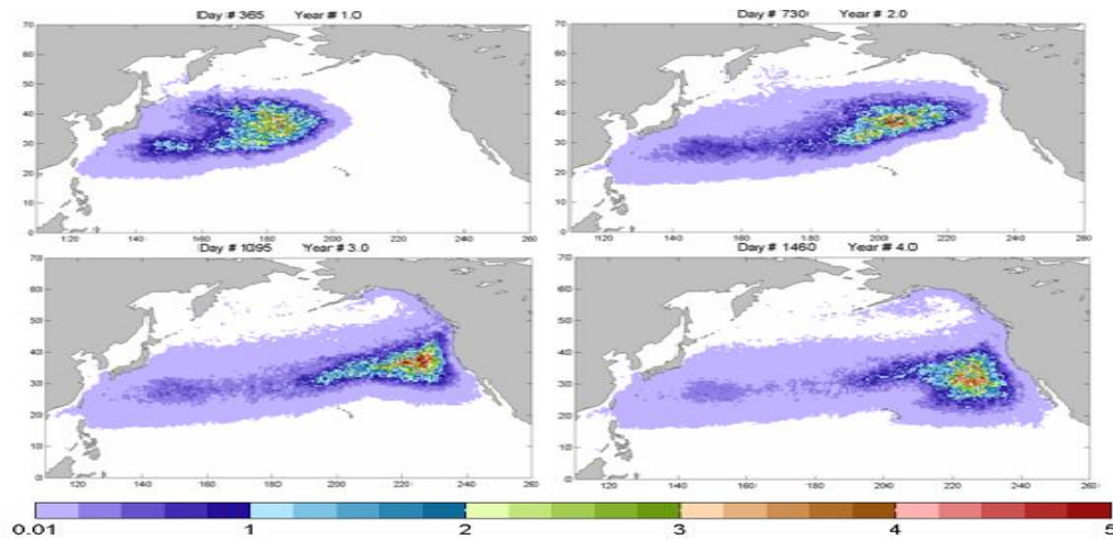
Gambar 5. Prediksi distribusi lepasan radionuklida ^{137}\text{Cs} di samudra Pasifik ( \text{Bq.L}^{-1} ) [3]
