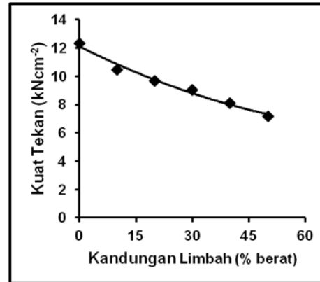
Gambar 8. Pengaruh Kandungan Limbah Terhadap Kuat Tekan Blok Polimer-NH 4 Zeolit Bekas.
