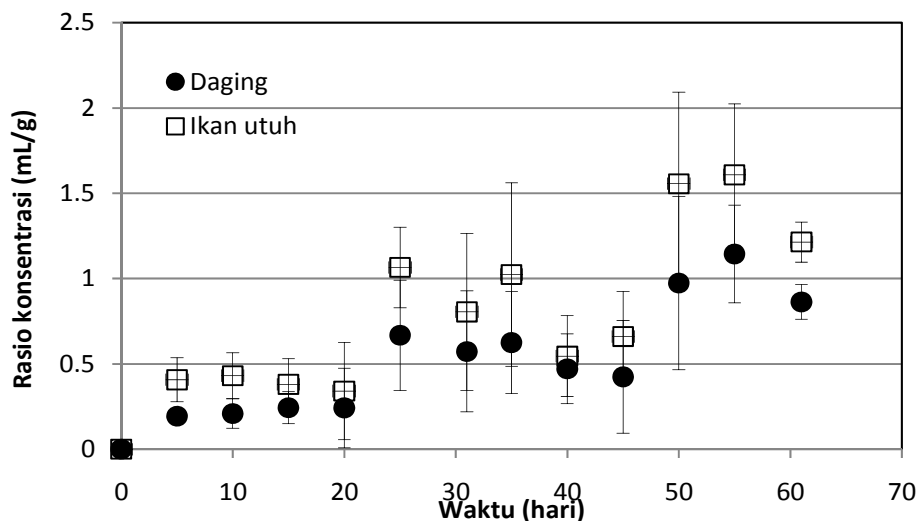
Gambar 6. Rasio konsentrasi ^{60}\text{Co} dalam tubuh ikan.
