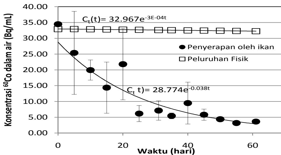
Gambar 4. Konsentrasi ^{60}\text{Co} dalam air sebagai fungsi waktu.
