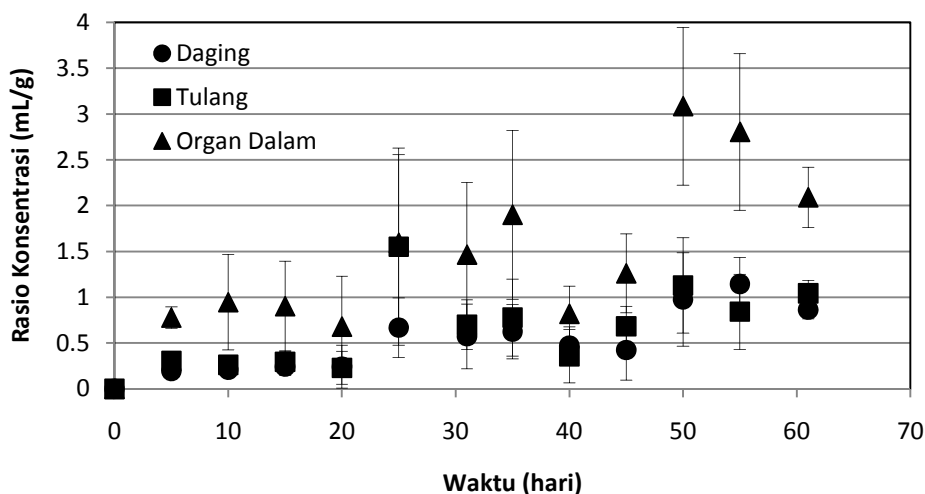
Gambar 5. Distribusi rasio konsentrasi ^{60}\text{Co} dalam bagian tubuh ikan.
