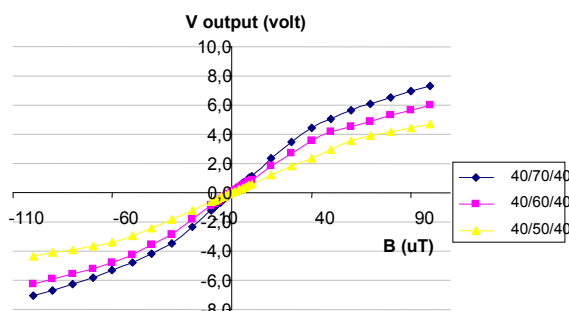
Gambar 12. Respon sensor terhadap variasi jumlah lilitan kumparan sekunder (pick-up coil)
