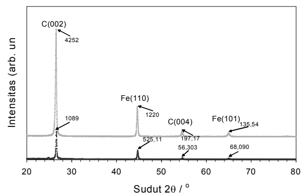
Gambar 3. Pola difraksi sinar-X material komposit Fe-C (—) sebelum dan (—) sesudah iradiasi sinar gamma pada dosis 250 kGy.
