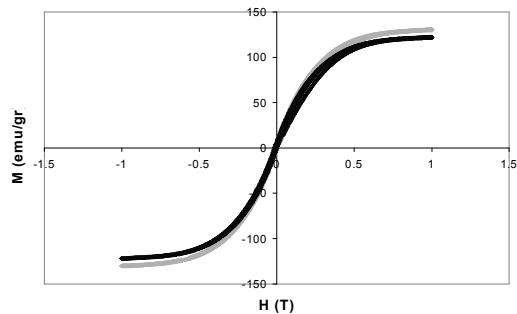
Gambar 6. Kurva magnetisasi Fe-C sebelum (—) dan sesudah (—) iradiasi pada dosis 250 kGy
