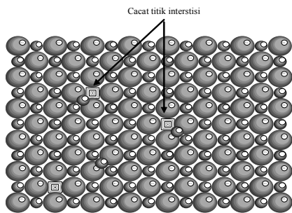
Gambar 4. Cacat titik interstisi yang terjadi pada struktur karbon/grafit oleh iradiasi sinar gamma.
