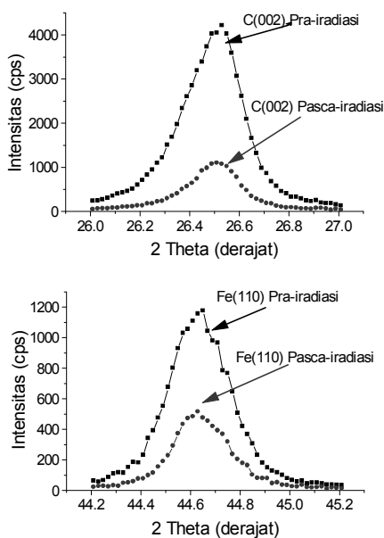
Gambar 5. Grafik hasil analisis data XRD dengan program origin untuk C [002] dan Fe [110] sebelum dan sesudah iradiasi sinar gamma
