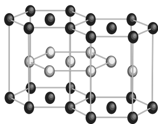
Gambar 1. Struktur heksagonal grafit
