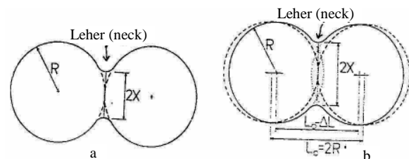
Gambar 3. a. Perpindahan permukaan ( surface transport ), b. Perpindahan muatan partikel ( bulk transport )
