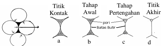
Gambar 1. a Bentuk titik kontak antar partikel serbuk dalam pelet mentah, b. Pembentukan awal batas butir, c. Pembesaran batas butir tahap pertengahan dan pengecilan pori, d. Bentuk batas butir pada akhir sintering
