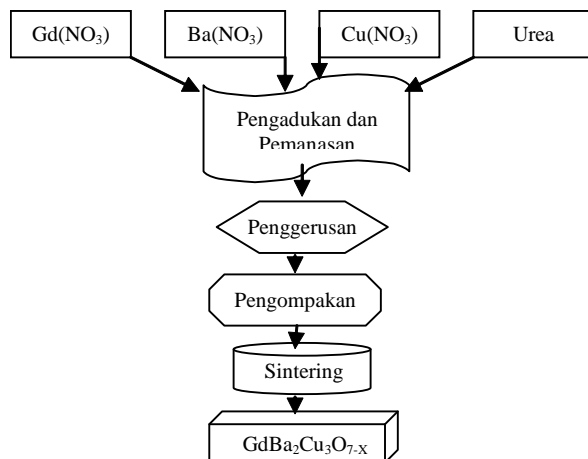
Gambar 3. Diagram alir pembuatan GdBa_2Cu_3O_{7-x}
