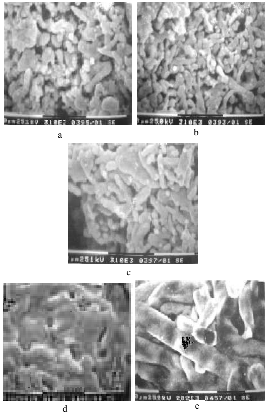
Gambar 5. Pertumbuhan morfologi GdBa_2Cu_3O_{7-x} pada sinter selama 5 jam dengan variasi suhu a. 800 °C, b. 850 °C, c. 900 °C, d. 925 °C dan e. 950 °C
