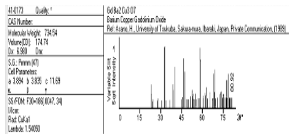
Gambar 7. Difraktogram standar GdBa_2Cu_3O_{7-x} dari JCPDS
