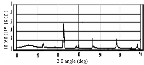
Gambar 9. Difraktogram sampel GdBa_2Cu_3O_{7-x} pada sinter 950 °C selama 5 jam.
