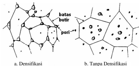
Gambar 2. Akibat ada densifikasi, Pori yang terdapat pada ujung batas butir (a), Pori yang terisolasi dalam butir (b).
