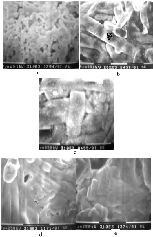
Gambar 6. Pertumbuhan morfologi GdBa_2Cu_3O_{7-x} pada suhu sinter 950 °C dengan variasi waktu a. 1 jam, b. 5 jam, c. 10 jam, d. 15 jam dan e. 20 jam
