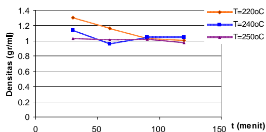
Gambar 6. Pengaruh waktu reaksi terhadap densitas produk.
