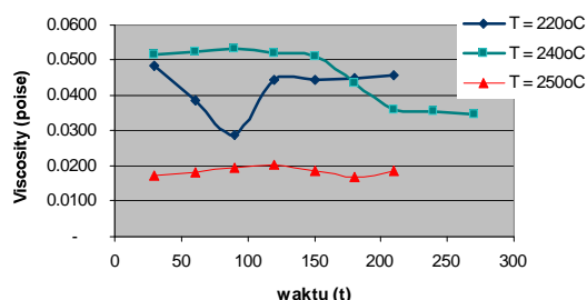
Gambar 4. Pengaruh Waktu Reaksi Pada Viskos
