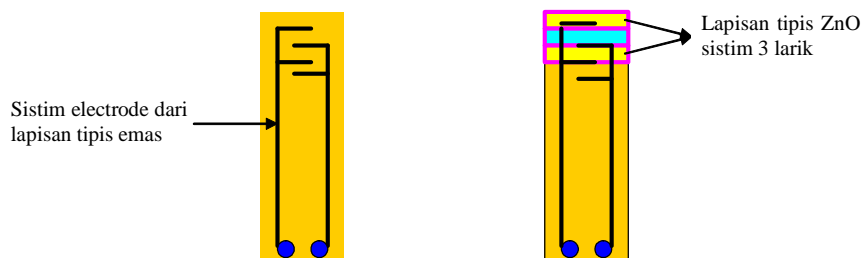
Gambar 2. Skema (a) sistim elektroda bagian depan dan (b) sistim lapisan tipis ZnO pada substrat Alumina ( Al_2O_3 ) bagian depan.
