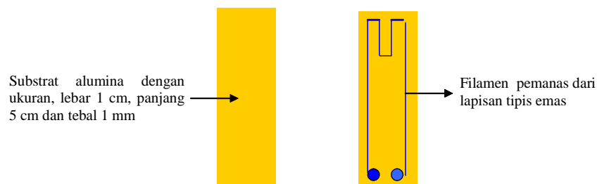
Gambar 1. Skema sistim pemanas pada substrat Alumina ( Al_2O_3 ) bagian belakang.
