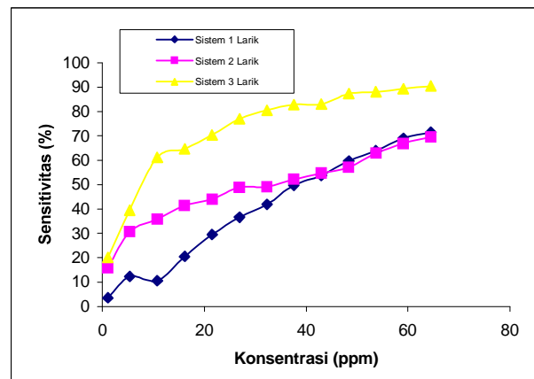
Gambar 4. Hubungan antara sensitivitas sensor ZnO sistem larik terhadap konsentrasi gas C 2 H 5 OH.
