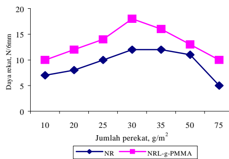
Gambar 5. Pengaruh jumlah perekat terhadap daya rekat antara focsing dengan kanvas.
