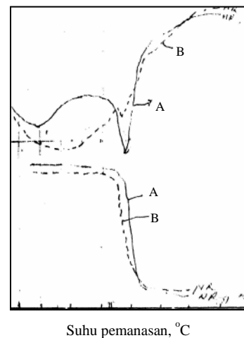
Gambar 10. Grafik DTA-TG NRL-g-MMA (A) dan kompon lateks alam vulkanisasi belerang (B).
