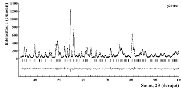
Gambar 2. Profil pola difraksi hasil analisis dengan metode Rietveld pada cuplikan fasa hijau Y-211 dengan asumsi parameter suhu anisotropis. Faktor R : R_{wp} = 9,29 ; R_p = 6,85 ; S = 1,03 ; R_l = 1,29 ; R_F = 0,73 . Parameter kisi : a = 12,184(3) Å, b = 5,662(1) Å, c = 7,135(2) Å. Volume sel satuan V = 492,3(2) Å 3 , kerapatan D = 6,132 g/cm 3 .
