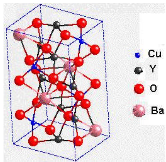
Gambar 3. Sel satuan fasa hijau Y_2BaCuO_5 , dimana lingkaran-lingkaran yang paling besar : ion Ba^{2+} ( r = 1,45 \text{ \AA} ) dan lingkaran paling kecil : ion Cu^{2+} ( r = 0,65 \text{ \AA} ), lingkaran terbesar kedua : O^{2-} ( r = 1,40 \text{ \AA} ) dan Y^{3+} ( r = 0,95 \text{ \AA} ).
