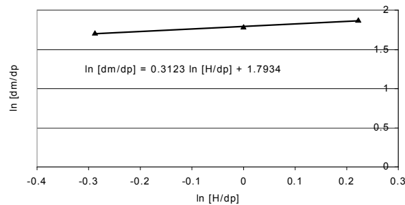
Gambar 3. Hubungan antara tinggi cairan dari dasar tangki terhadap ukuran microsphere terbentuk.
