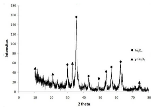
Gambar 1. Spectra XRD nanopartikel Fe_3O_4
