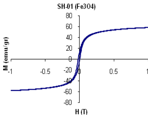
Gambar 2. Magnetisasi nanopartikel Fe_3O_4
