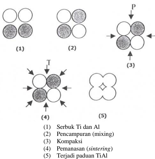
Gambar 1. Tahapan pemaduan proses metalurgi serbuk.
