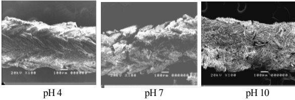
Gambar 1. Foto SEM dengan perbesaran 100 kali dari benang bedah Polyglactin 910 sebelum dan setelah inkubasi selama 4 minggu dan 9 minggu dalam berbagai pH.
