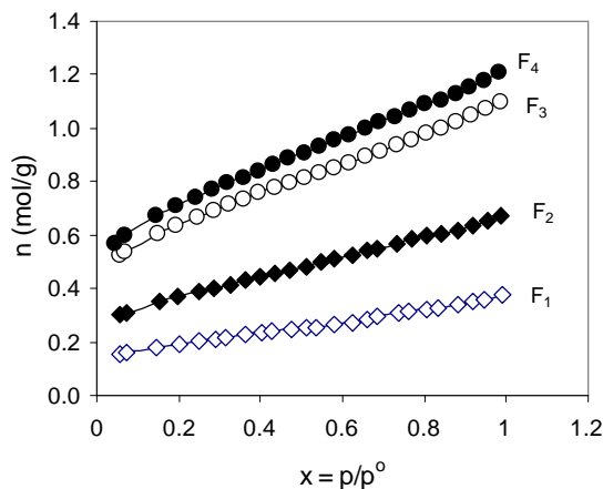
Gambar 4. Adsorpsi isothermal nitrogen pada fraksi bentonit.
