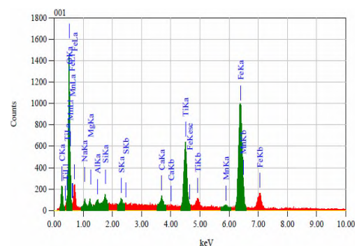
Gambar 1. Analisis elementer menggunakan EDS sampel pasir besi hasil separator magnetik
