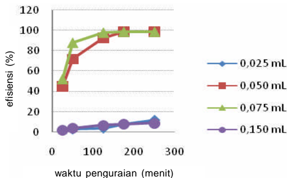
Gambar 7. Pengaruh konsentrasi H 2 O 2 dan waktu penguraian terhadap efisiensi degradasi MB dengan metode fenton untuk Fe 3 O 4 (Aldrich).
