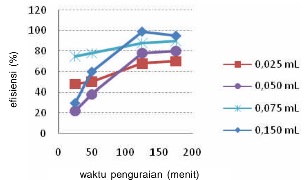
Gambar 8. Pengaruh konsentrasi H 2 O 2 dan waktu penguraian terhadap efisiensi degradasi MB dengan metode foto fenton untuk Fe 3 O 4 (Aldrich).
