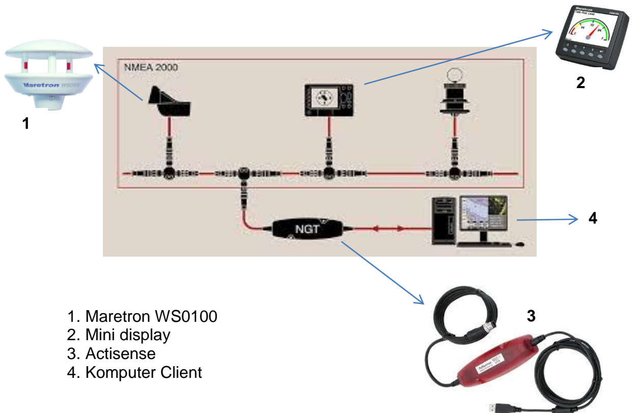
Gambar 3 Komunikasi antara sensor Maretron WS0100 dengan komputer client
