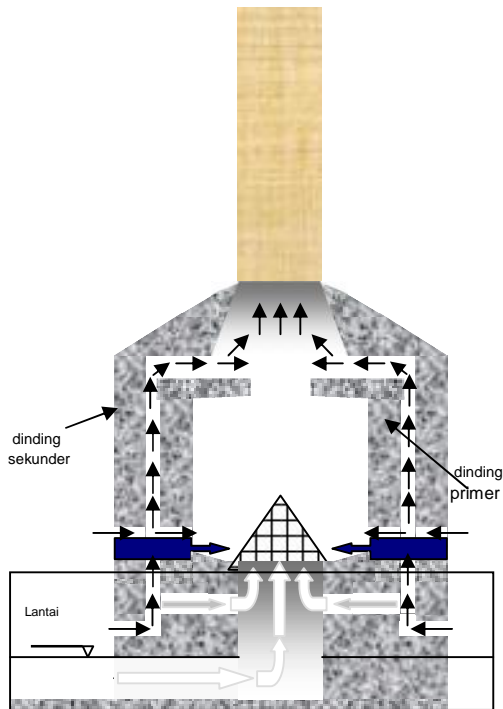
Gambar 7. Irisan Vertikal Tungku
