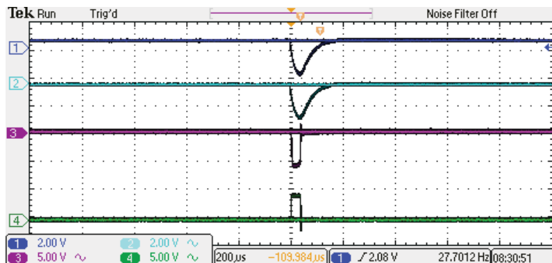
Gambar 8. Keluaran Modul Sistem Deteksi Radiasi Untuk Detektor GM
