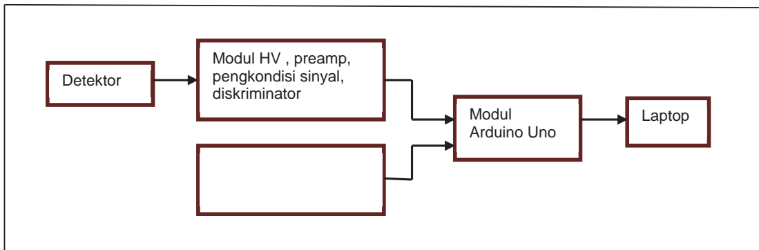
Gambar 6. Blok Diagram Pengujian Sistem Deteksi Monitor Lingkungan
