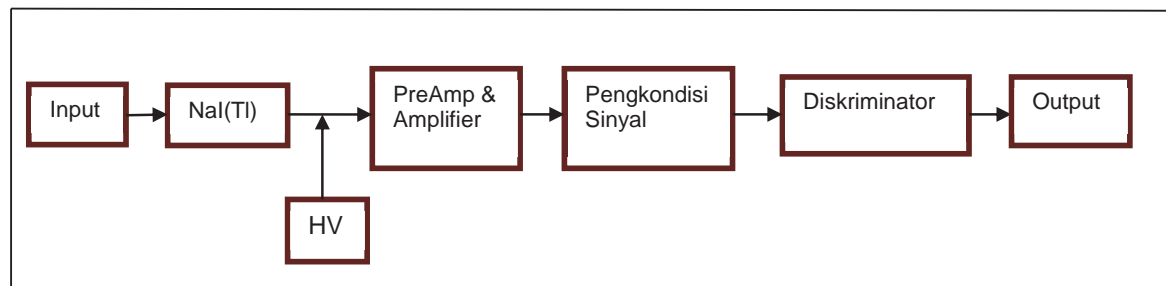
Gambar 2. Blok Diagram Sistem Deteksi Radiasi Menggunakan Detektor NaI(Tl)
