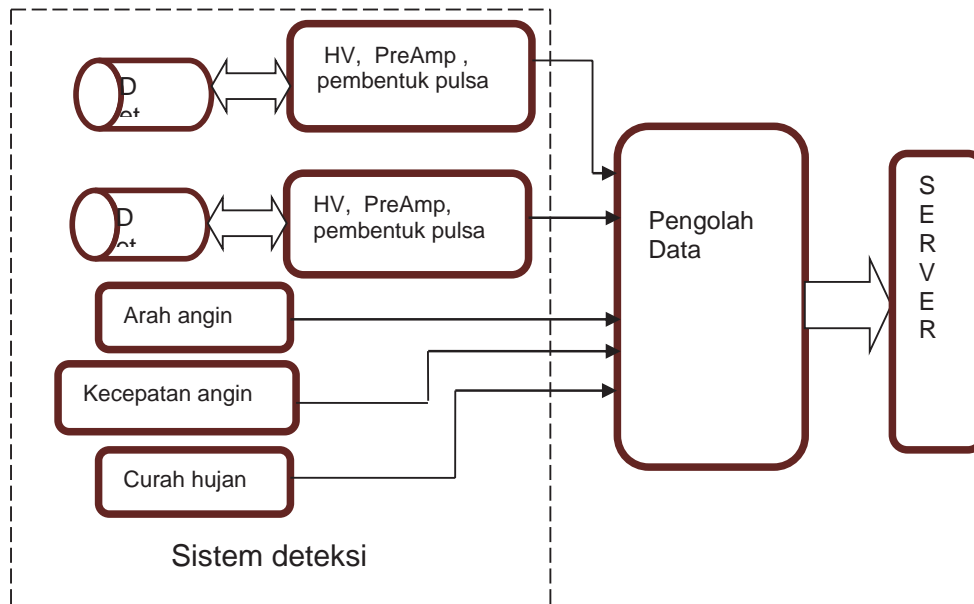
Gambar 1. Sistem Pemantau Radioaktifitas Lingkungan
