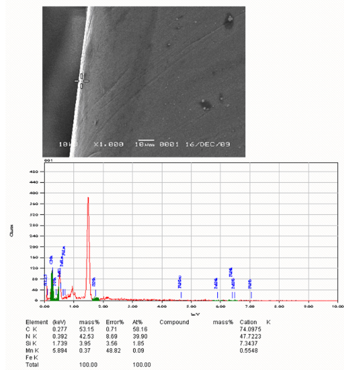
Gambar 6. Mikrograf SEM-EDAX dari tampang-lintang pena piston pada proses nitridasi ion: waktu nitridasi 4 jam, suhu nitridasi 100 °C dan tekanan gas nitrogen 1,6 mbar.
