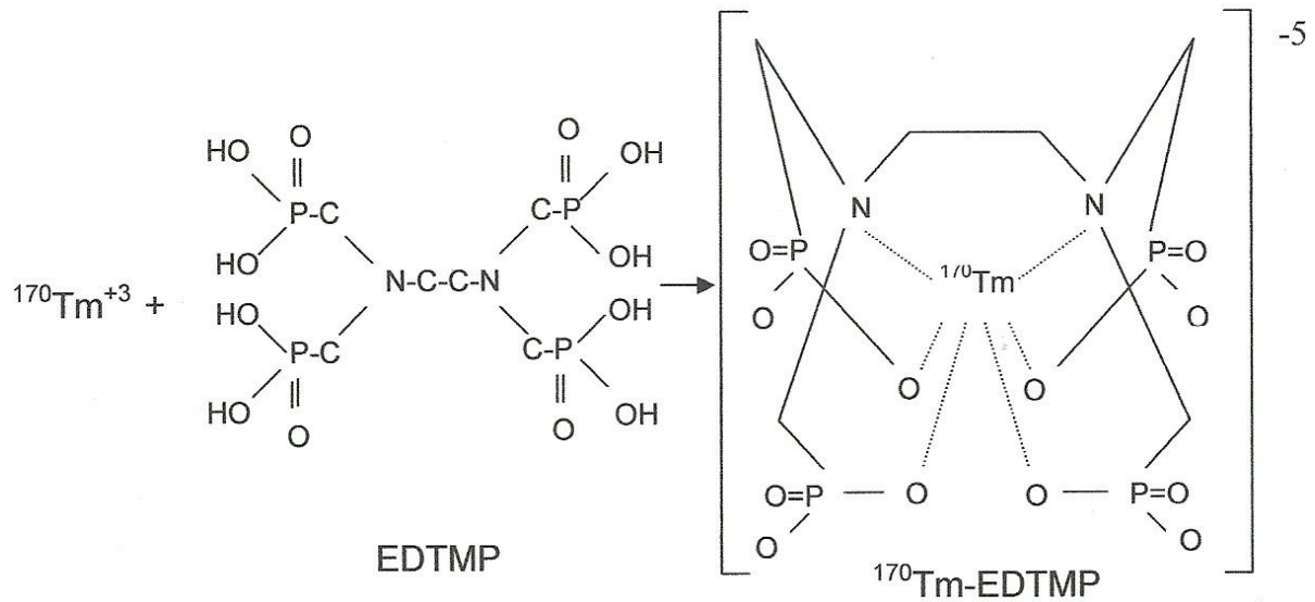
Gambar 3. Struktur kimia senyawa kompleks ^{170}\text{Tm-EDTMP}
