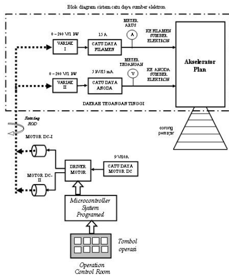
Gambar 10. Blok Diagram Sistem catu daya sumber elektron
