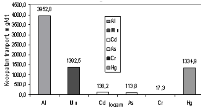
Gambar 4. Kecepatan transpor logam di dalam arus air sungai Kancilan
