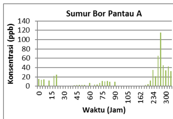
Gambar 10. Grafik konsentrasi rhodamin terhadap waktu (jam) pada SBP-A.
