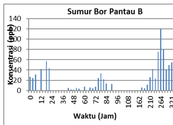
Gambar 9. Grafik konsentrasi rhodamin WT terhadap waktu (jam) pada SBP-B.
