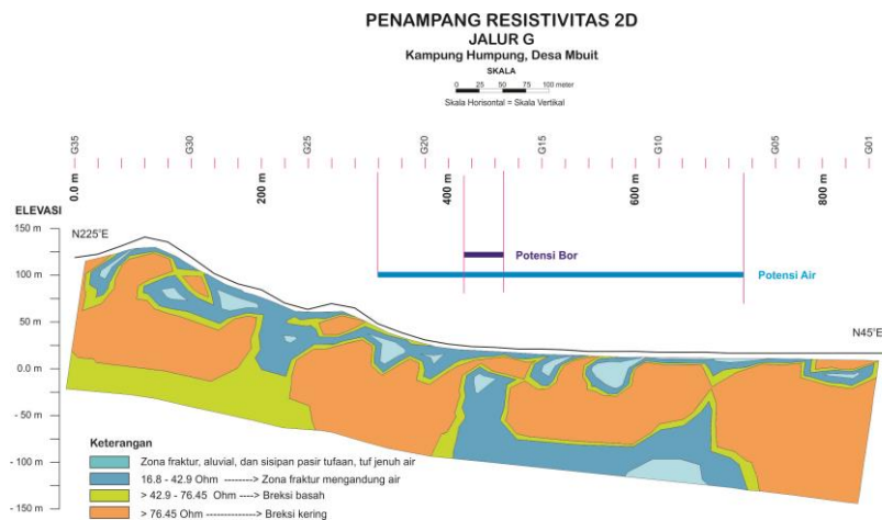
Gambar 11. Penampang resistivitas dua dimensi Lintasan G, Desa Mbuti, Kecamatan Bolong.
