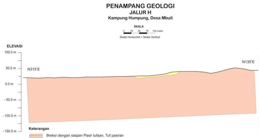
Gambar 17. Penampang geologi hasil interpretasi resistivitas 2D Jalur H, Desa Mbuit, Kecamatan Boleng.
