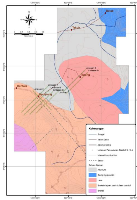
Gambar 7. Peta lintasan pengukuran geolistrik di Desa Mbuti, Kecamatan Bolong.
