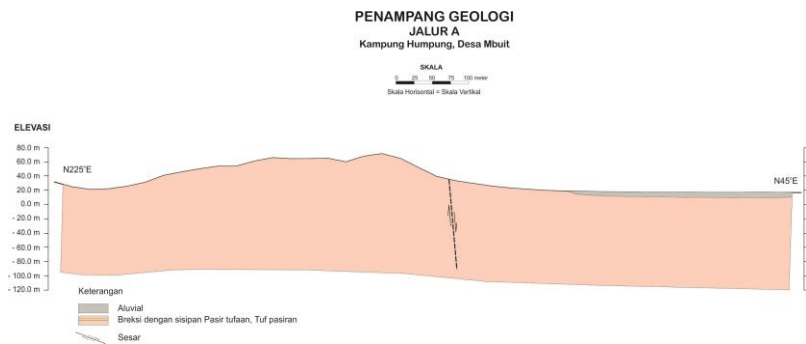
Gambar 13. Penampang geologi hasil interpretasi resistivitas 2D Jalur A, Desa Mbuti, Kecamatan Boleng.
