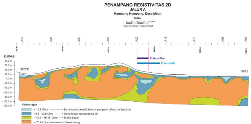
Gambar 8. Penampang resistivitas dua dimensi Lintasan A, Desa Mbuti, Kecamatan Bolong.
