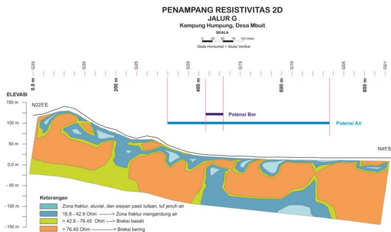
Gambar 11. Penampang resistivitas dua dimensi Lintasan G, Desa Mbuti, Kecamatan Bolong.
