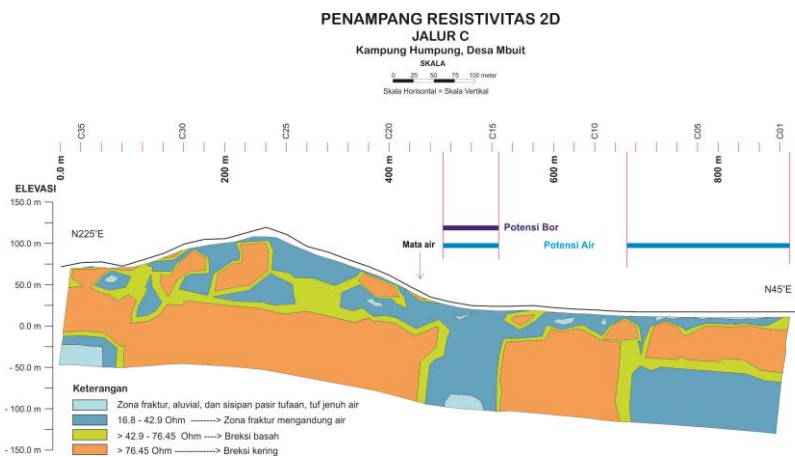
Gambar 10. Penampang resistivitas dua dimensi Lintasan C, Desa Mbuti, Kecamatan Bolong.
