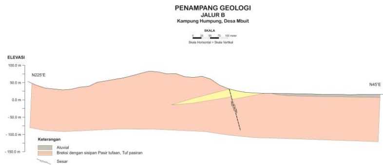
Gambar 14. Penampang geologi hasil interpretasi resistivitas 2D Jalur B, Desa Mbuti, Kecamatan Boleng.
