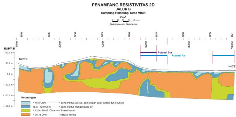
Gambar 9. Penampang resistivitas dua dimensi Lintasan B, Desa Mbuti, Kecamatan Bolong.
