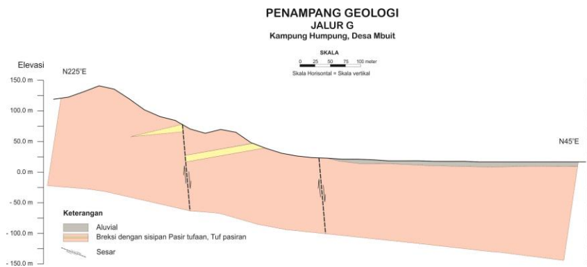
Gambar 16. Penampang geologi hasil interpretasi resistivitas 2D Jalur G, Desa Mbuti, Kecamatan Boleng.
