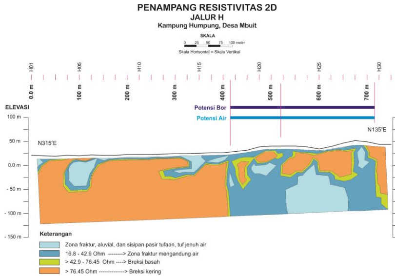
Gambar 12. Penampang resistivitas dimensi Lintasan H, Desa Mbuti, Kecamatan Boleng.
