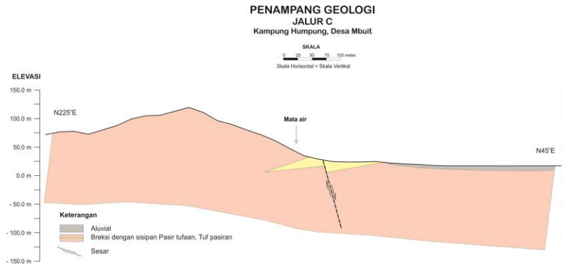
Gambar 15. Penampang geologi hasil interpretasi resistivitas 2D Jalur C, Desa Mbuti, Kecamatan Boleng.
