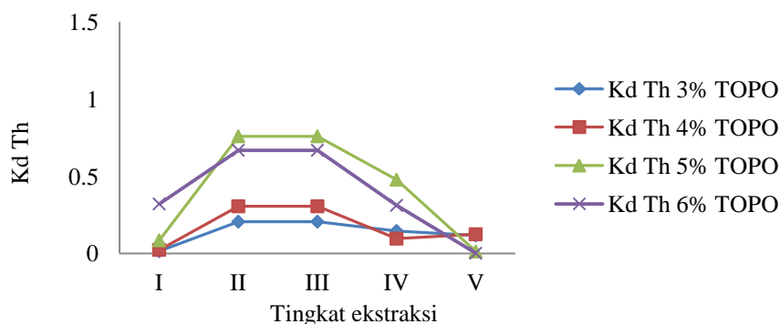
Gambar 5. Hubungan antara tingkat ekstraksi Th pada berbagai % TOPO–Kerosen.
