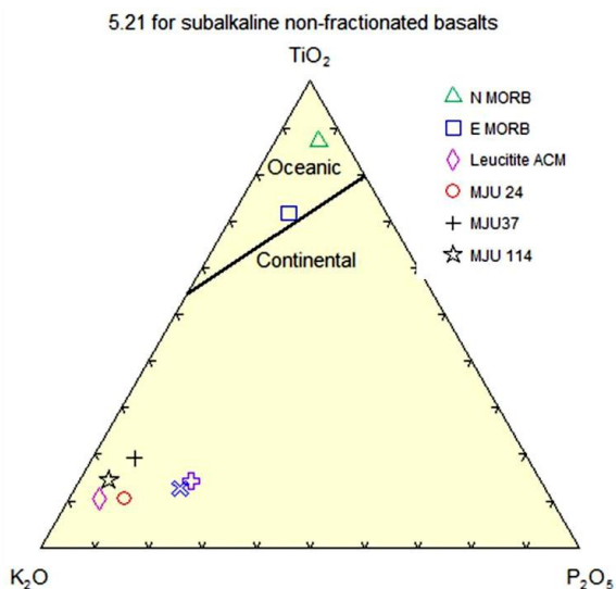
Gambar 8. Hasil plot pada diagram K_2O-P_2O_5-TiO_2 [15].
