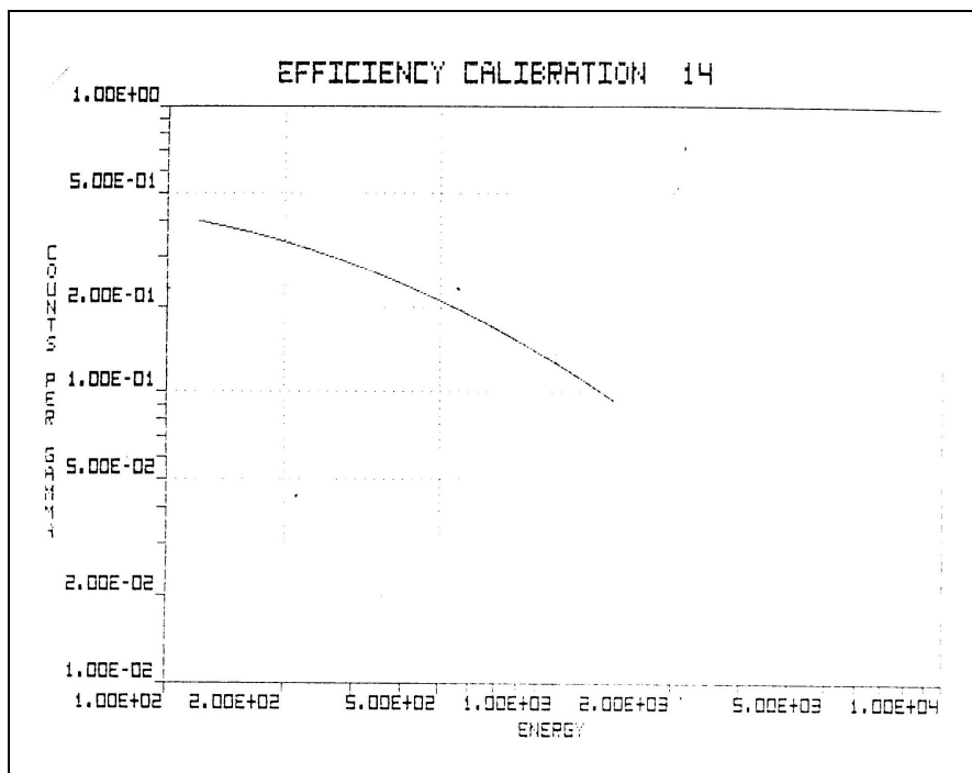
Gambar 2. Kurva Kalibrasi Efisiensi detektor HpGe alat cacah WBC ACCUSCAN-
