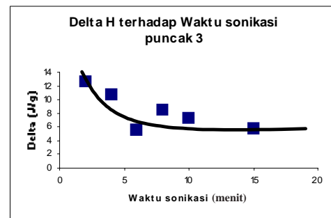
Gambar 8. Penurunan entalpi pada puncak pelelehan PLA.
