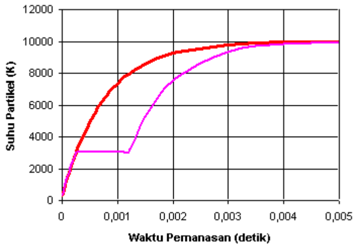
Gambar 7. Suhu partikel YSZ bentuk bola berdiameter 50 μm dalam plasma jet bersuhu 10000K sebagai fungsi waktu pemanasan tanpa dan dengan proses pelelehan.
