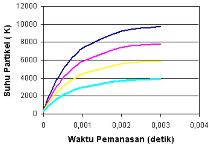
Gambar 6. Kurva pemanasan partikel YSZ berukuran 50 μm sebagai fungsi waktu pemanasan dengan berbagai variasi suhu plasma jet 10000,8000, 6000 dan 4000 K
